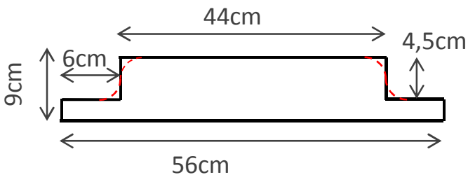
Schéma 7: empiècement
