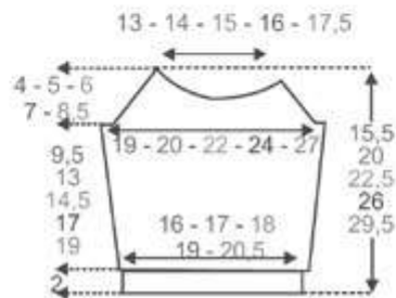
Patron manche droite
